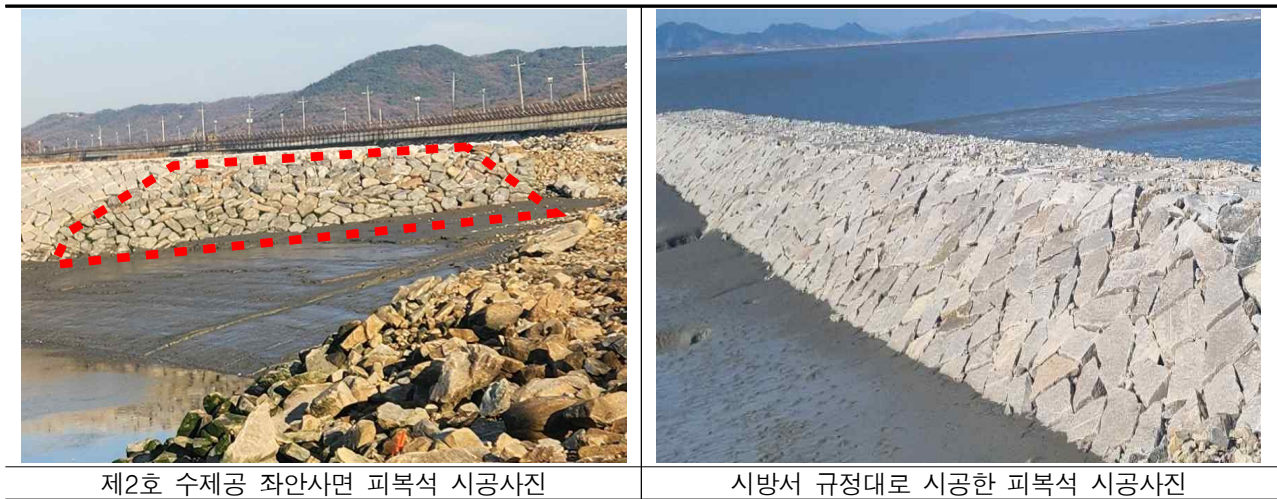
[그림 2] 피복석 시공 상태
